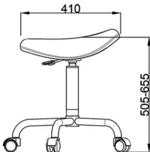
Maßzeichnung
