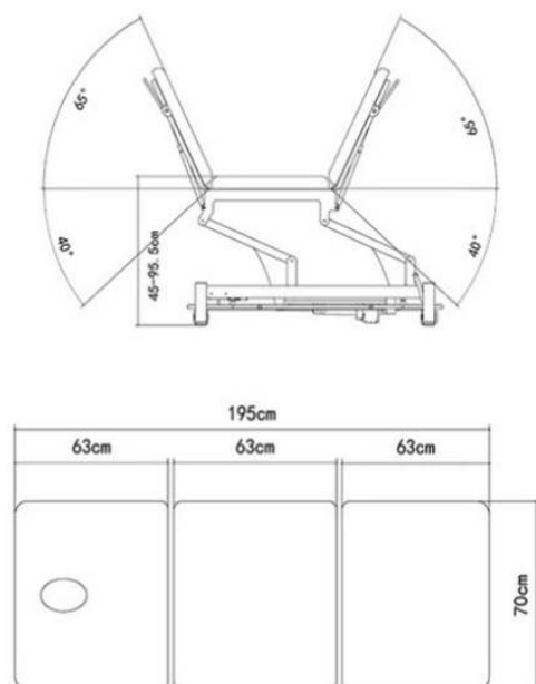
Maßzeichnung
